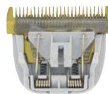
79000 02 / Tête de coupe < 46 mm >
